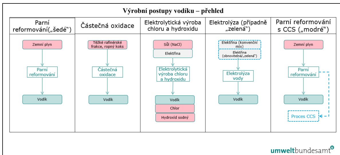
Obrázek 5-3: Hranice systému různých výrobních postupů vodíku – přehled
